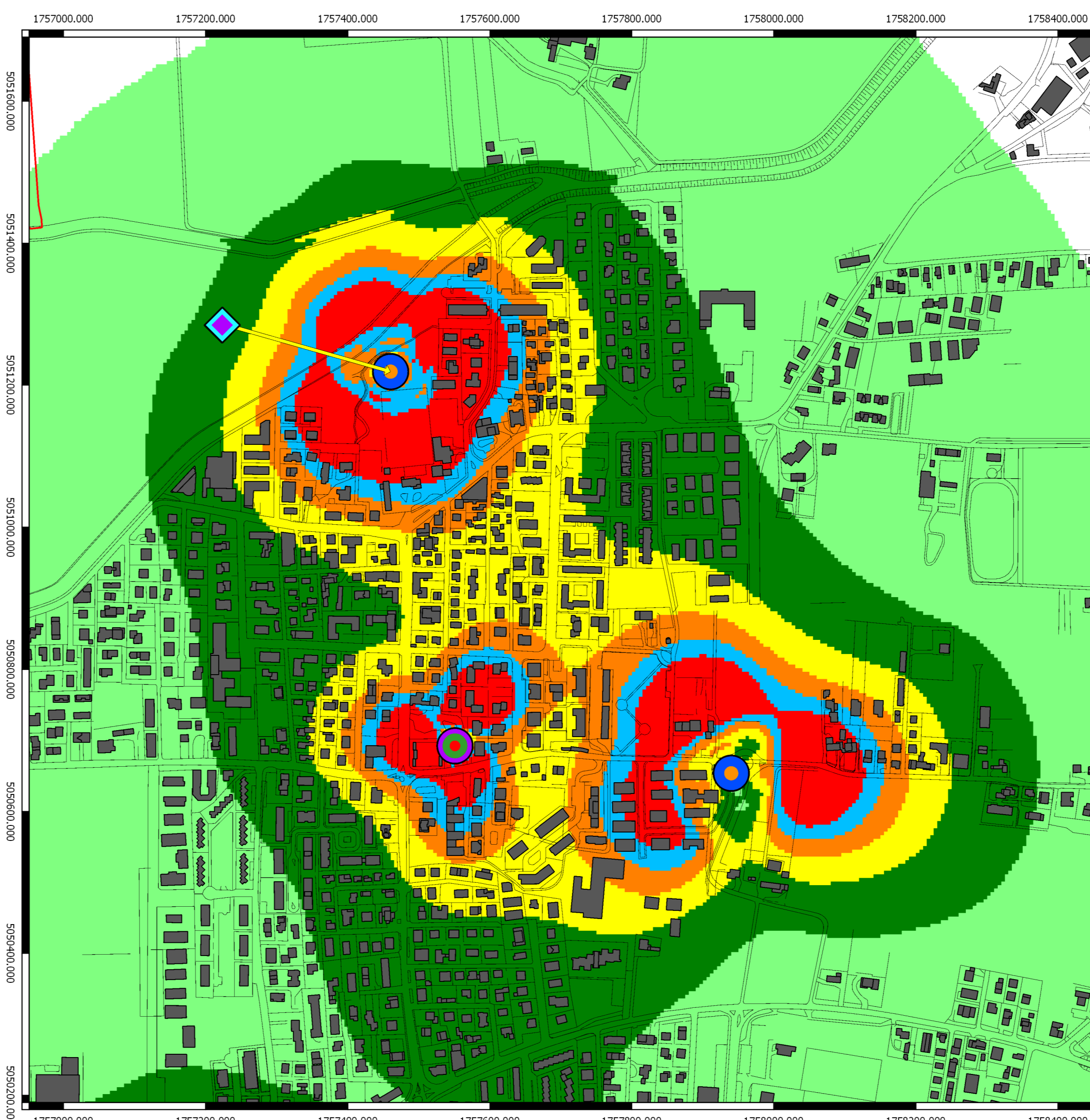
Campo elettromagnetico (V/m) calcolato alla quota di 17,5 m sul livello del terreno
