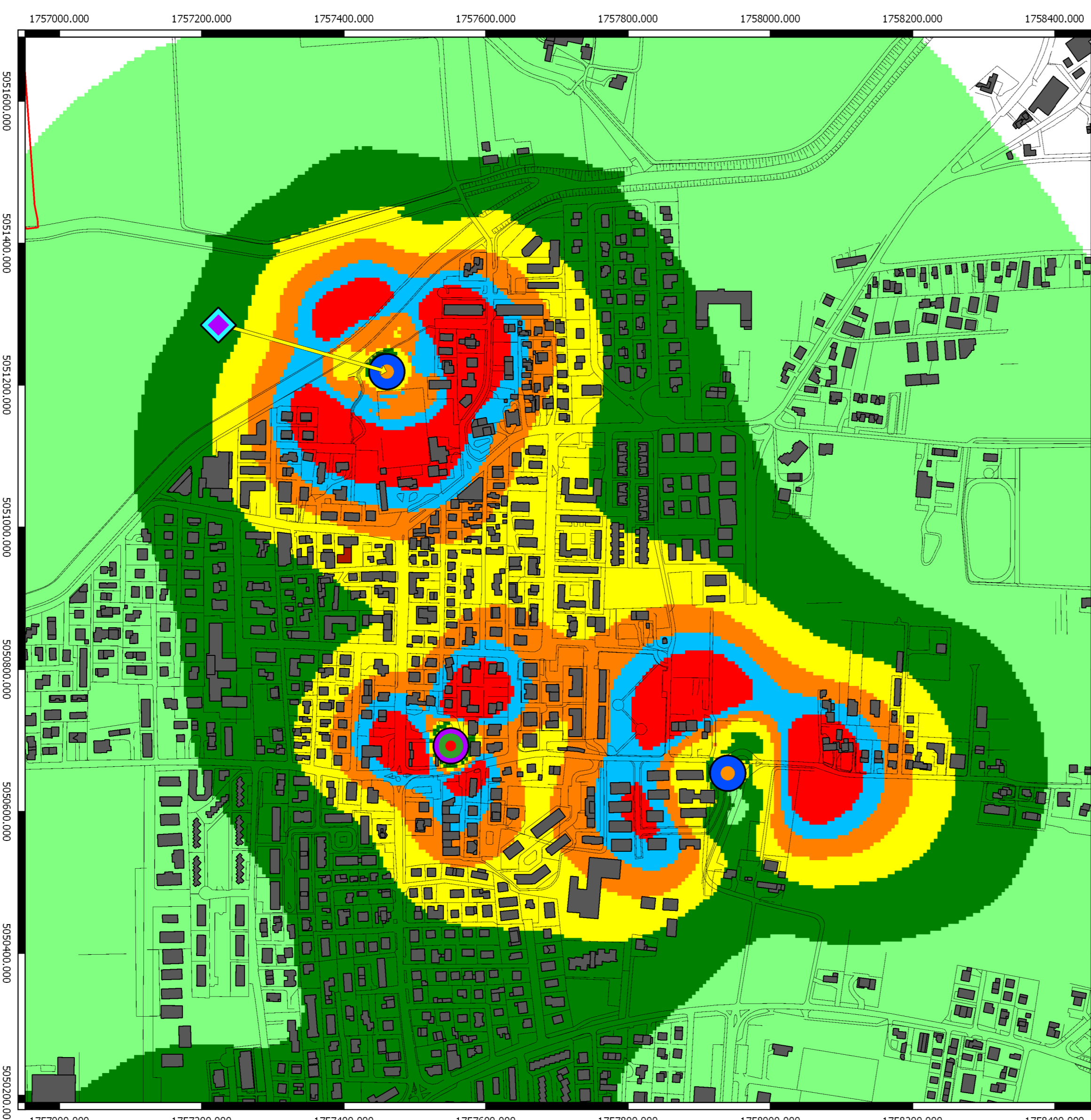
Campo elettromagnetico (V/m) calcolato alla quota di 15,5 m sul livello del terreno
